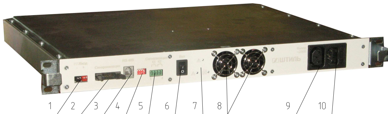
Рисунок 1.3 - Инвертор Штиль PS48-60/1000
